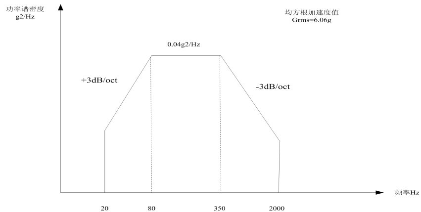
图 2 随机振动功率谱密度图
