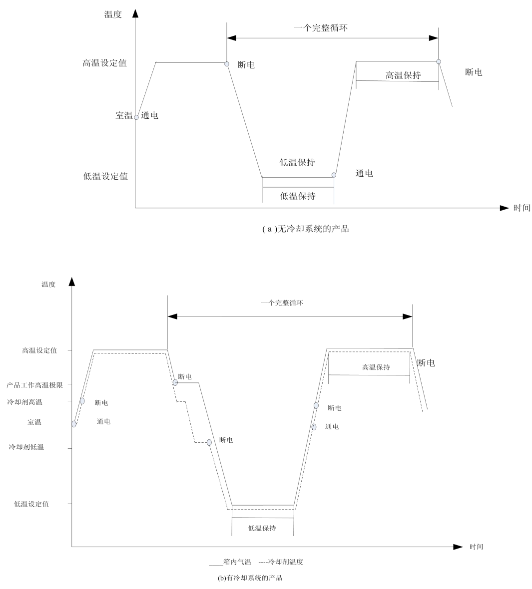
图 1 温度循环图
