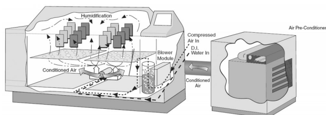
Q-FOG®CRH 循环腐蚀盐雾箱可进行相对湿度控制
