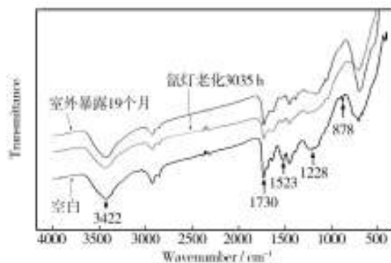
图3 三亚室外自然曝晒和氙灯老化后聚氨酯涂层红外光谱图
