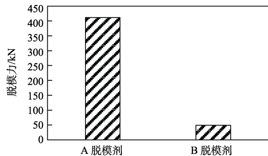
图 6 A、B 脱模剂脱模力对比
